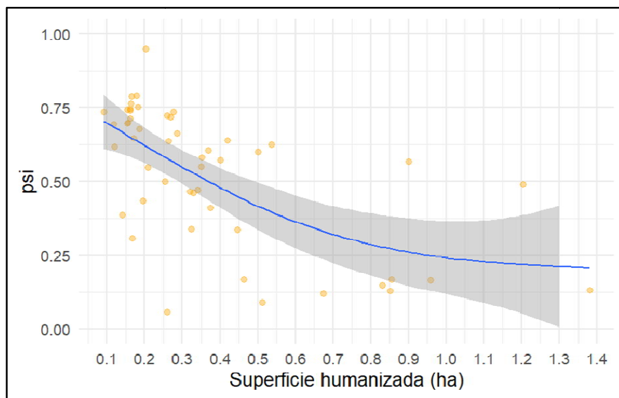
Figura 11. Datos predictivos de probabilidad de ocupación en función de las variables que destacan en el mejor modelo: Superficie humanizada. (Brinzal)
